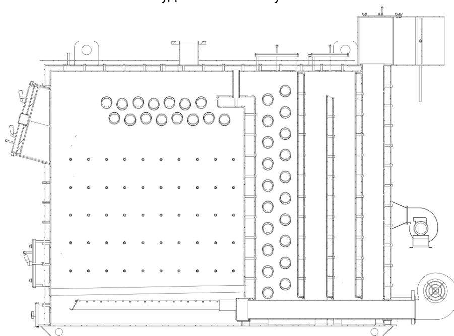
Рис.3в Будова котлів потужністю 1250кВт:
