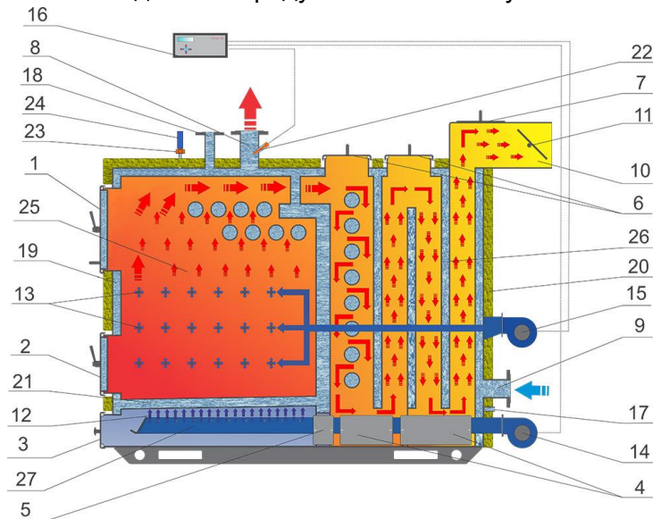
Рис.3 Будова котлів модельного ряду «Retra-3M» потужністю 250-2000кВт
