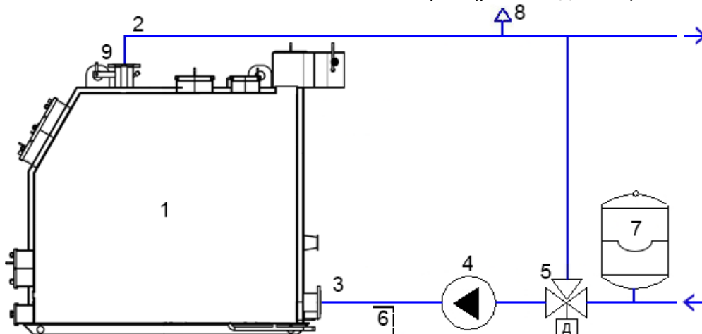
Рис.7 Схема об'язки котла з бойлером (рекомендована)
