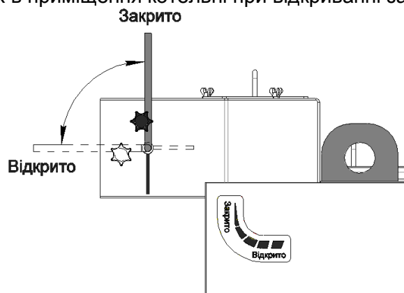
Рис.10 Схема налаштування шибера димоходу в положення (ЗАКРИТО-ВІДКРИТО)
